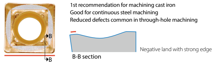
Tough edge: GH chipbreaker
